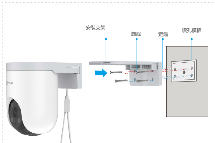
圖 2 壁掛式安裝
